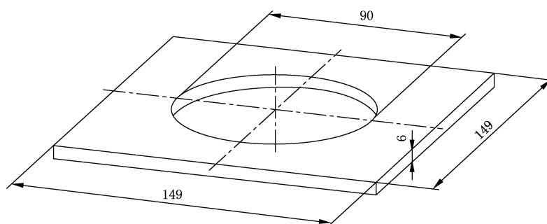
图 B.4 热量计定位板
