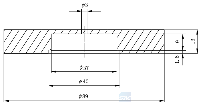
图 B.2 热量计安装台
